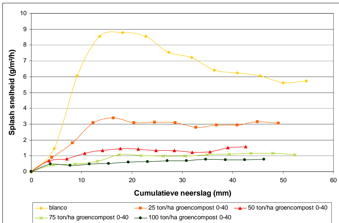
Figuur 11 Evolutie van de splash snelheid in functie van de cumulatieve neerslag bij de regenvalsimulaties. 33
